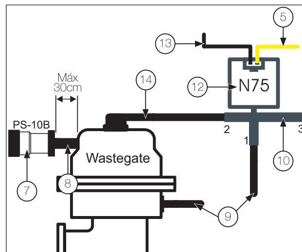
Diagrama con Válvula N75
