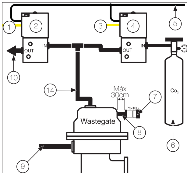
Diagrama con solenoides
