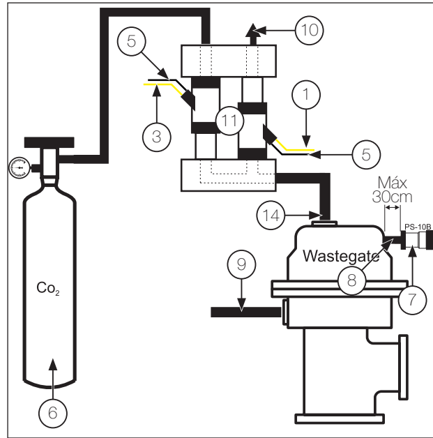
Diagrama con Válvula 3 vías
