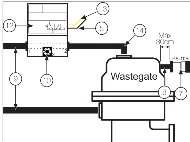
Diagrama con Válvula 3 vías
